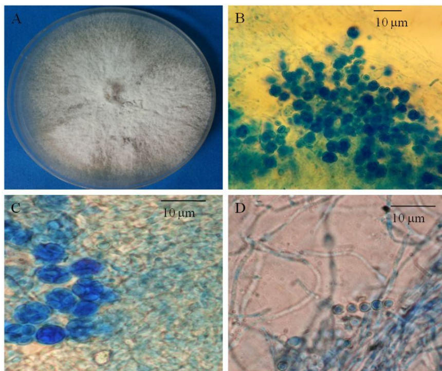
شکل 2- گونه Byssochlamys nivea : (A) پرگنه هفت روزه روی محیط کشت PDA، (B-C) آسک و آسکوسپورها و (D) کنیدیوم‌ها
